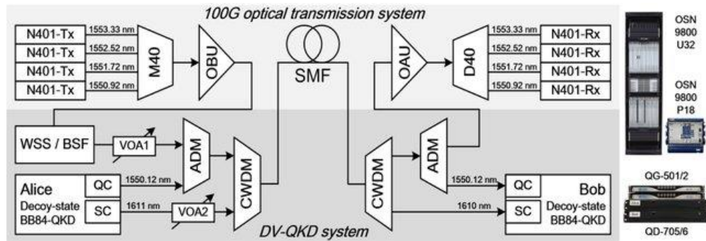
2.5. ábra – kvantum csatornát integráló rendszer elrendezése [11]
