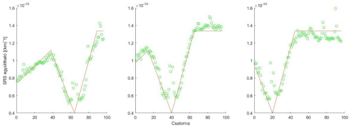
5.4. ábra – A fotonzámból SRS együtthatóvá átszámított mért értékek (zöld), és a módosított modell szerinti görbe (piros)
