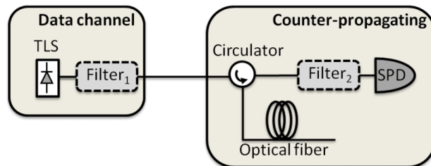
2.3. ábra – SRS szórodott foton detektáló mérési elrendezése [10]
