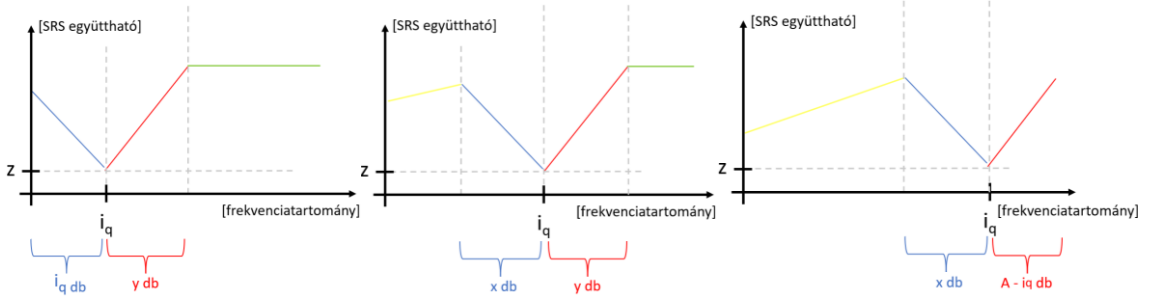
5.2. ábra – SRS együttható összegzésénél figyelembe vett 3 eset
