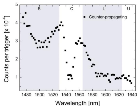
2.4. ábra – ellentétes irányú SRS mérésének eredménye [10]
