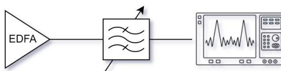
3.7. ábra – hangolható szűrő mérésének blokkváza
