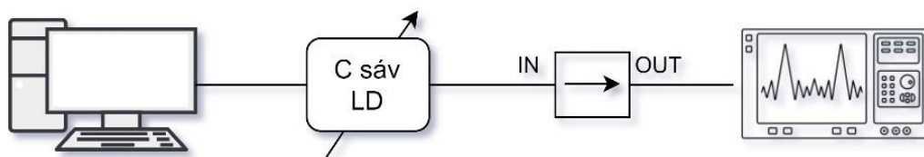
3.5. ábra – izolátor csillapításának mérésének blokkváza
