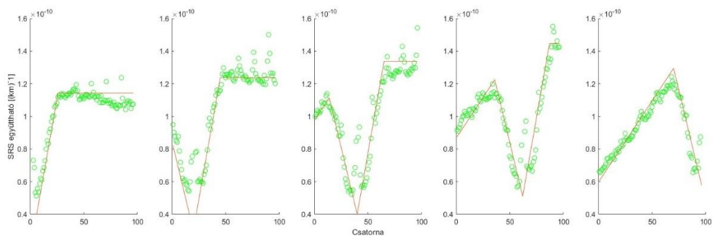
6.2. ábra – Az SRS együtthatóvá átszámolt mért értékek (zöld), és a pontosított z változóval korrigált modell szerinti görbe (piros)
