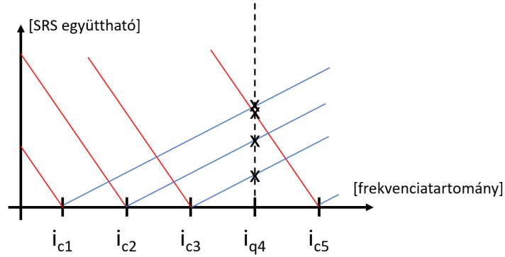
2.9. ábra – SRS együttható 5 csatornával szemlélítve
