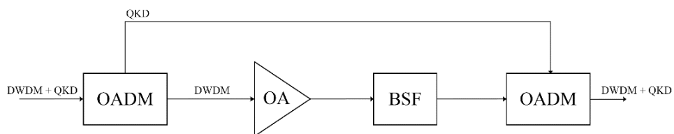
1.4. ábra – optikai erősítő kikerülése QKD-val (OADM: Optikai add-drop multiplexer, OA: optikai erősítő, BSF: sávzáró szűrő)
