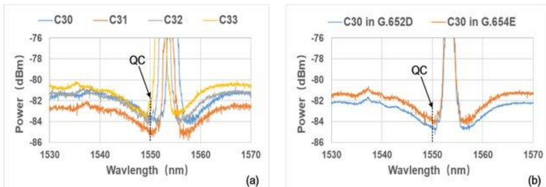
2.6. ábra – klasszikus csatornák SRS zajának teljesítménye, hullámhossz függvényében [11]
