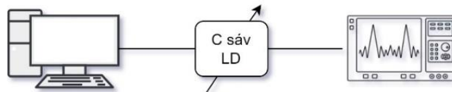
3.2. ábra – hangolható lézer mérésének blokkváza
