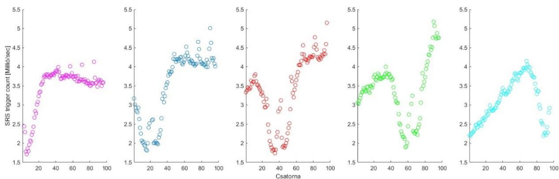
6.1. ábra – Sorrendben: 1. csatorna (rózsaszín), 20. csatorna (sötét kék), 40. csatorna (piros), 62. csatorna (zöld), 96. csatorna (világos kék)
